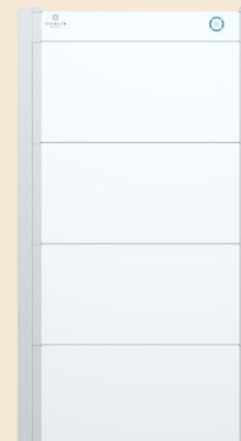
Stromspeicher SP-HE30727-H Hochspannung Lithium-Eisen-Phosphat- Batterie (LFP) Maximale Sicherheit, Lebensdauer und Leistung Gesamt Speicherkapazität: 8,29kWh Speicherkapazität jederzeit erweiterbar bis zu 55,3 kWh Schutzklasse: IP65 Maße(B/H/T): 640x1940x1220mm Gewicht: 96kg 10 Jahre Hersteller Garantie
